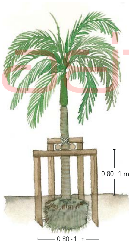
การค้ำยันแบบคอก
