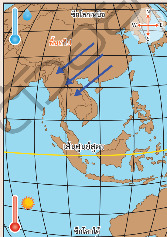
รูปที่ 8 ทิศทางลมในช่วงมรสุมตะวันออกเฉียงเหนือ
