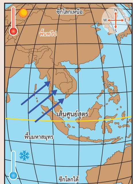
รูปที่ 7 ทิศทางลมในช่วงมรสุมตะวันตกเฉียงใต้
