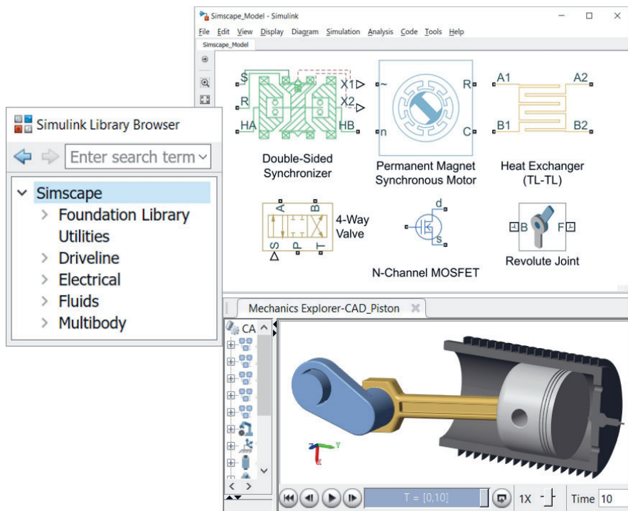
รูปที่ 2.20 MATLAB Simulink กับแบบจำลองด้าน Control Systems; Plant Dynamics
