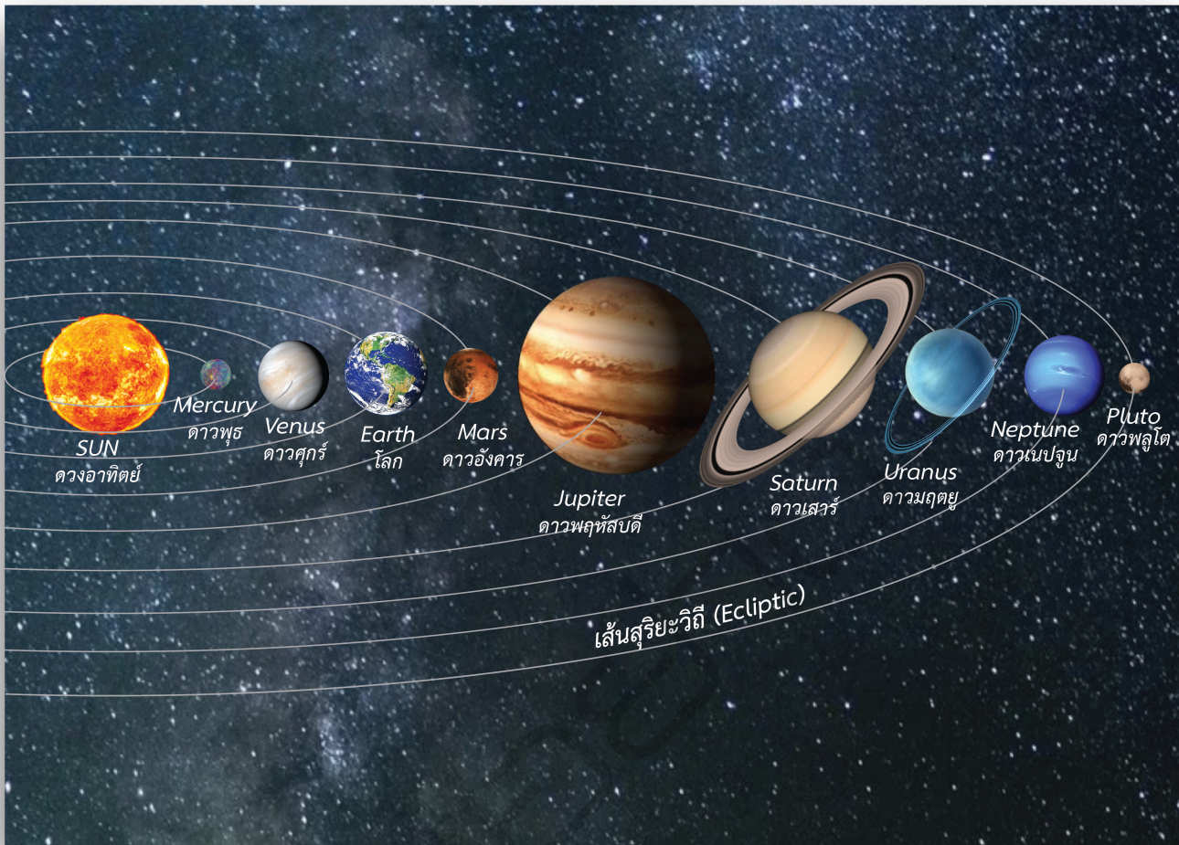
รูปที่ 1. แสดงระบบสุริยะ (Solar System)
