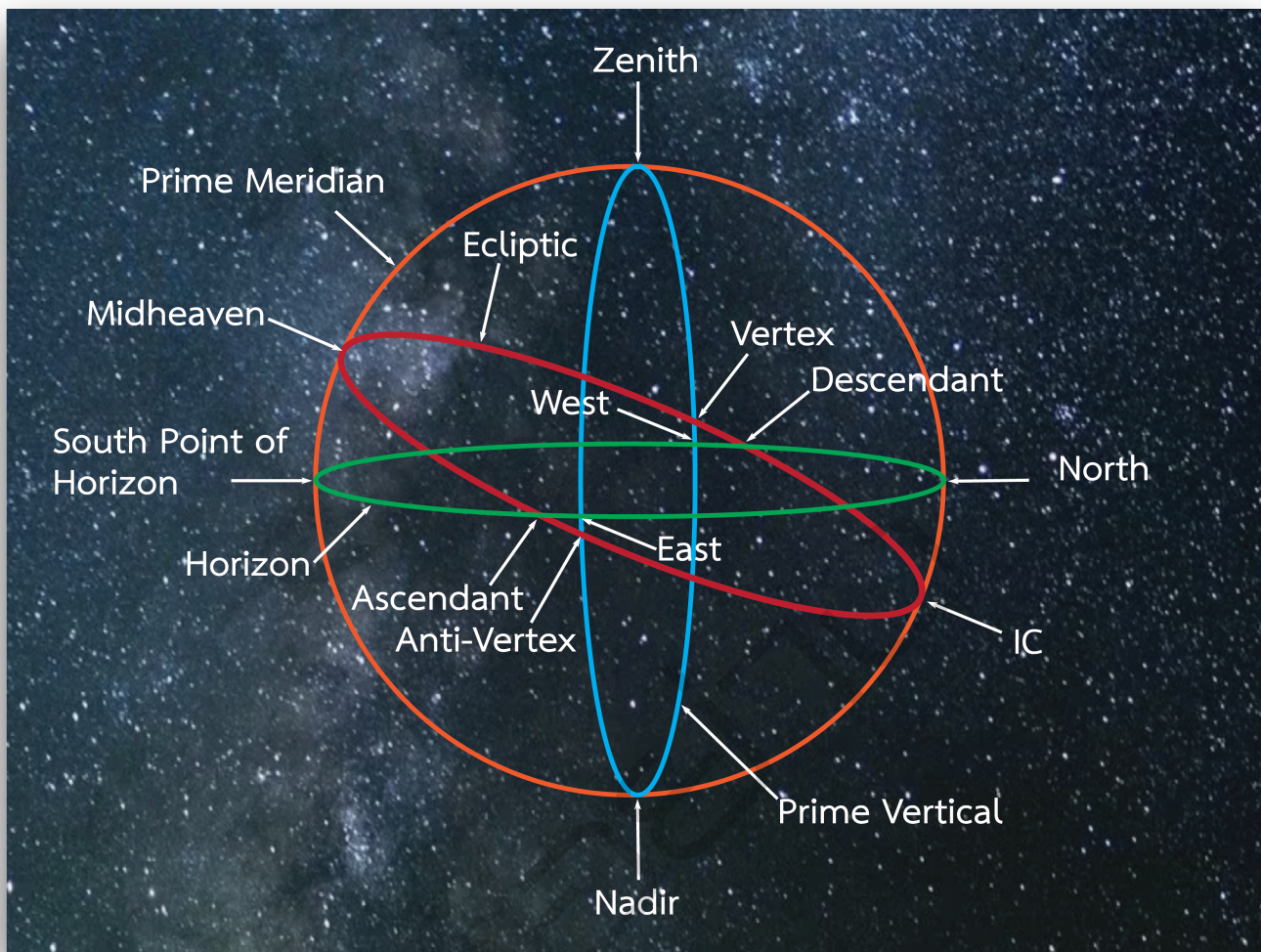
รูปที่ 3. แสดงที่มาของเส้น และจุดสำคัญต่างๆ
