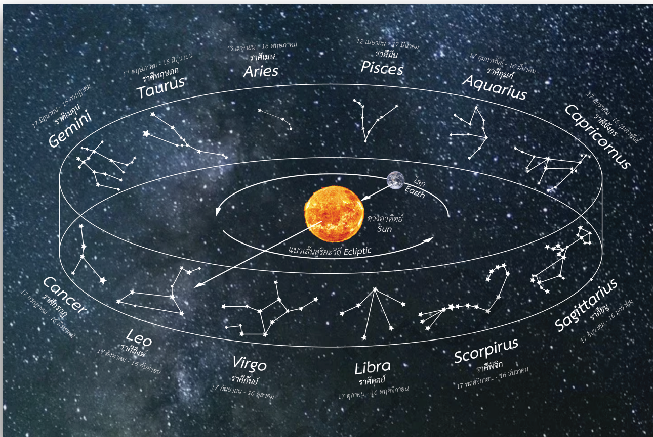
รูปที่ 2. ราศี(Zodiac)
