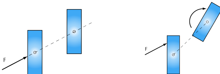
รูป 1.4 แรงกระทำที่ผ่านจุดศูนย์กลางมวลของวัตถุ วัตถุจะเคลื่อนที่โดยไม่หมุน
