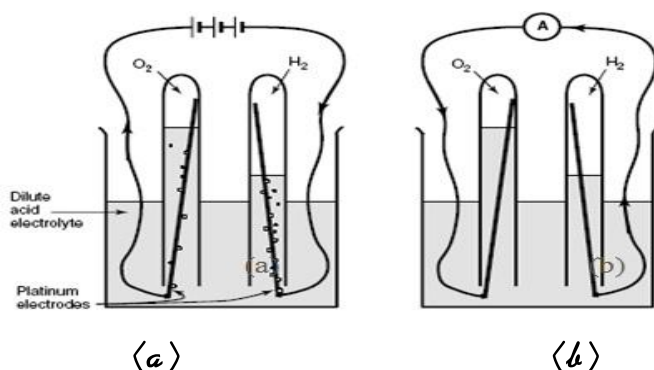
รูป 5 (a) กระแสไฟฟ้า ทำให้น้ำแยกออกเป็นไฮโดรเจนและออกซิเจน (b) การรวมกันของไฮโดรเจนและออกซิเจน จะได้กระแสไฟฟ้า
