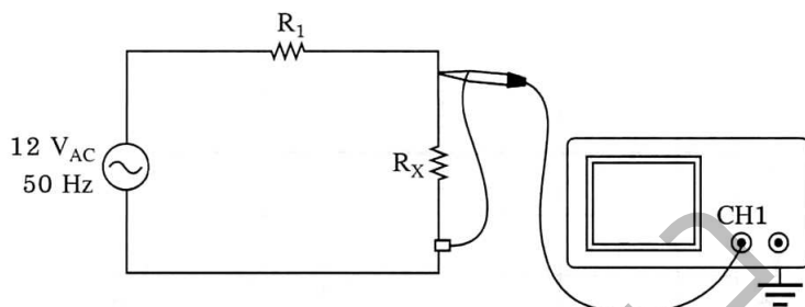
(ก) การใช้ออสซิลโลสโคปวัดแรงดันไฟสลัตกคร่อม R_x
